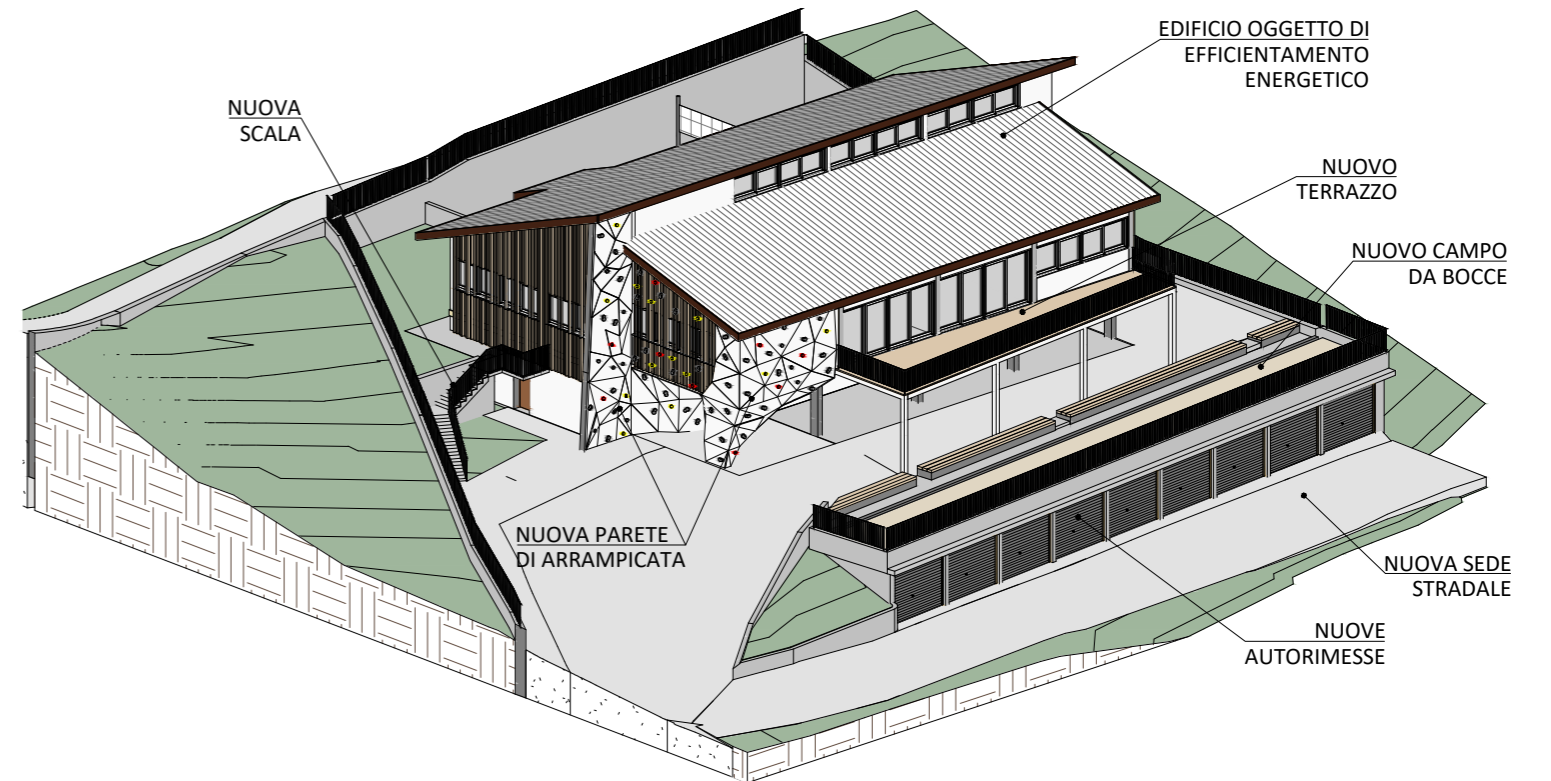
ASSONOMETRIA
